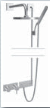
HANSAMATRIX функциональная часть- комплект инсталляции O3 однорычажный смеситель, DN 15 (G1/2) 4487 3030 хромиров. подходит для HANSASTELA- с комплектом душевой штанги- Верхний душ HANSARAIN DN 15
