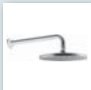
HANSAVIVA верхний душ, DN 15 4426 0100 хромиров. верхний душ, латунь Ø 200 мм выступ: 350 мм
