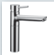
HANSAVANTIS STYLE Новинка однорычажный смеситель для умывальника, DN 15 с приподнятым цоколем 5247 2203 хромиров. 5242 2273 хромиров. ручка карандаш. сливной гарнитур и управление толкателем (сбоку), Подключение через гибкие шланги G 3/8 выступ: 216 мм
